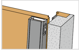
Gâche plate
